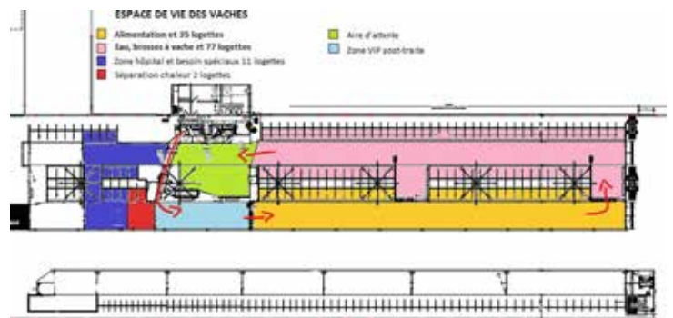
Plan d'étable en circulation semi-guidée.
